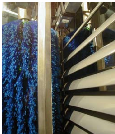
Es handelt sich hierbei um ein stationäres Reinigungssystem, das nach dem Prinzip der Bürstenwalzenreinigung horizontale Innen- und Außenjalousien sämtlicher Größen reinigen kann.
